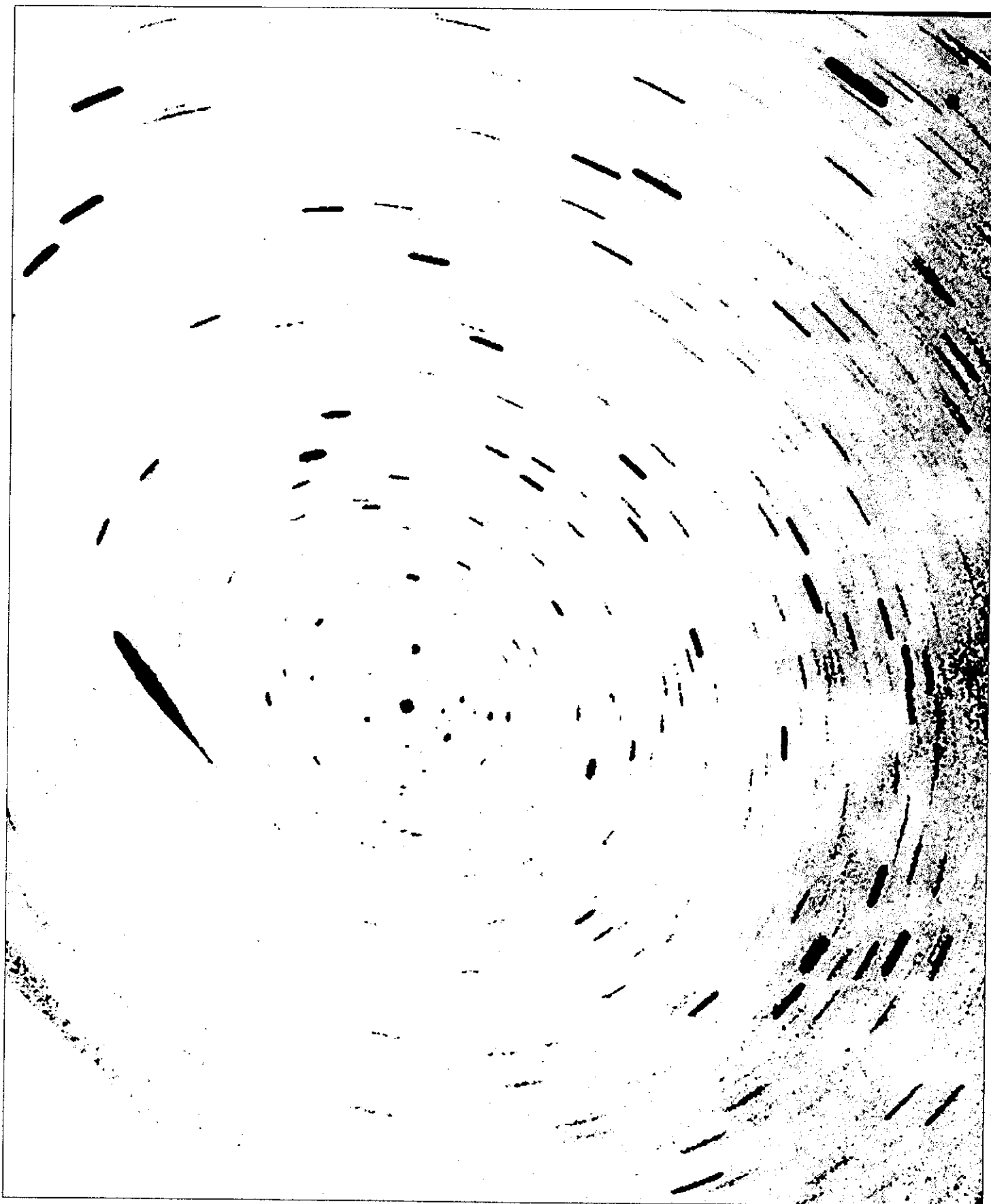
Obr. 3 - Meteor z roje Perseid nad Coloradem v USA. Fotografoval Vic Winter na film Kodak Ektapress 1600, 20 minutovou expozicí dne 12. srpna 1994. Podle Astronomy December 1994 zpracoval RAM.
